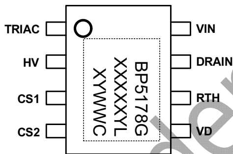
图2 管脚封装图
